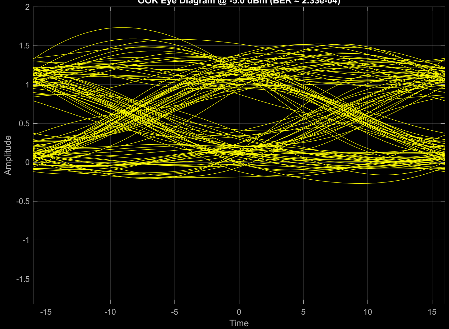
OOK Eye Diagram @ -5.0 dBm (BER \approx 2.33\text{e-}04 )
